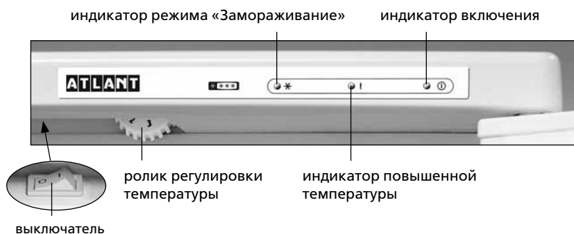
Рисунок 3 – Органы управления морозильника
