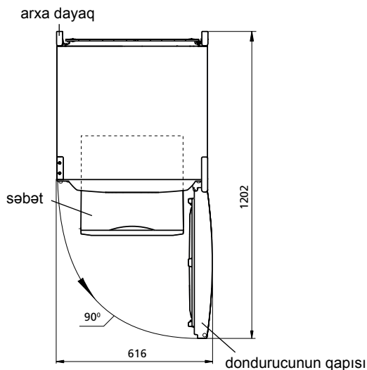
Şəkil 2 – Dondurucu (yuxarıdan görünüş)
