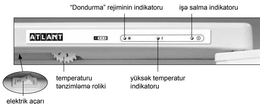
Şəkil 3 – Dondurucunu idarəetmə orqanları
