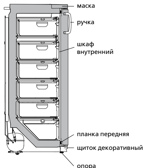
Рисунок 6 – Схема морозильника
